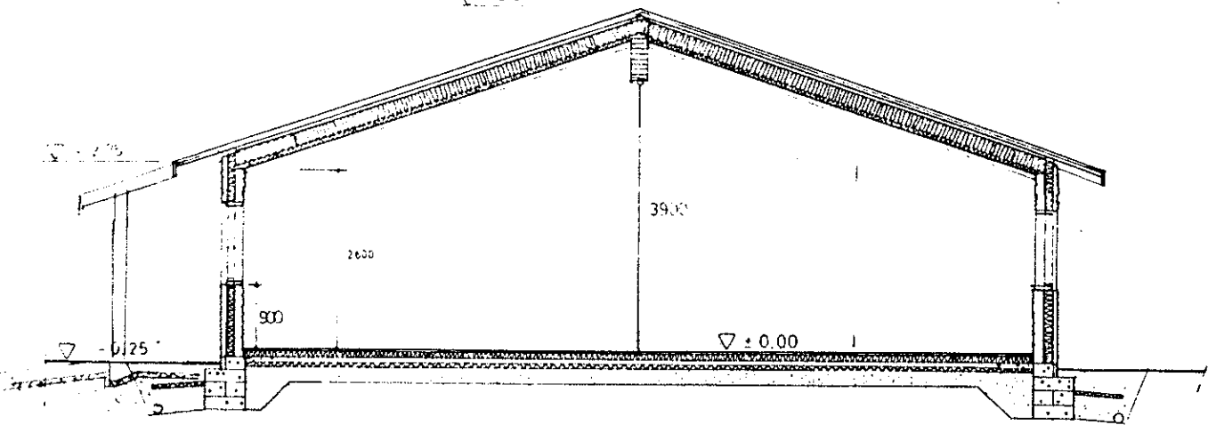
LEIKKAUS A-A
