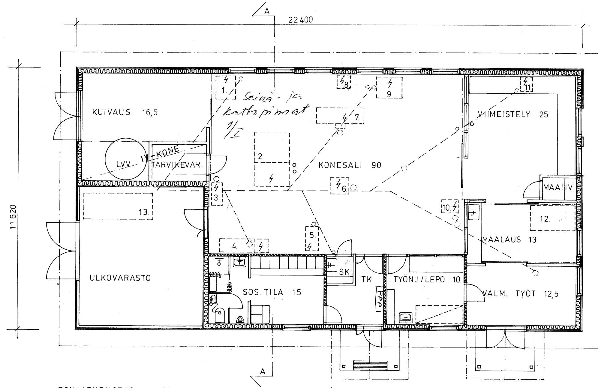
POHJAPIIRUSTUS 1:100
