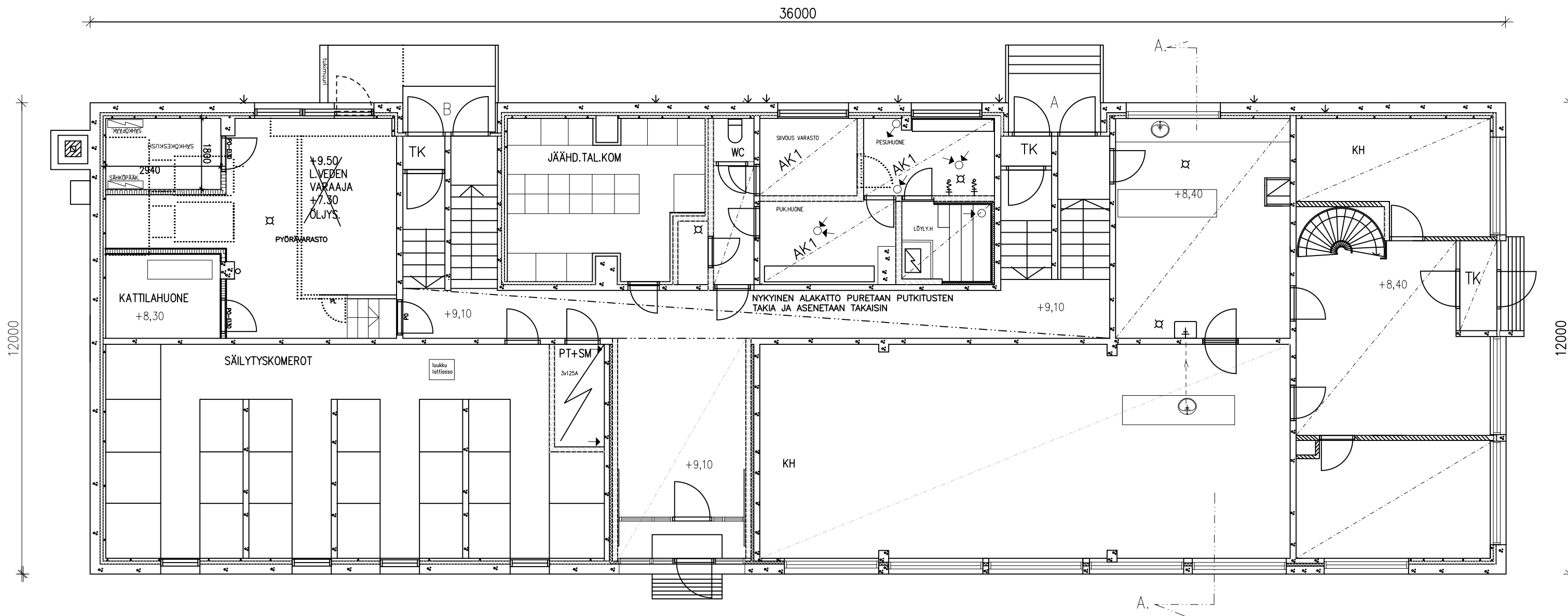
YLÄKELLARI 1:100
