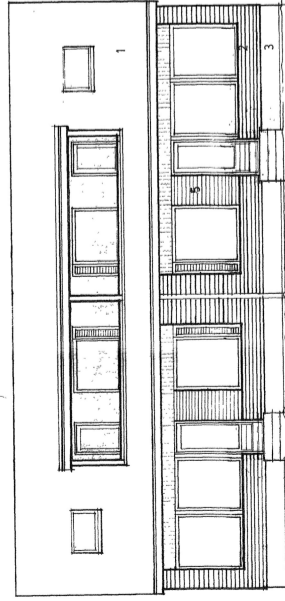
SIVU ETELÄÄN 1:100
