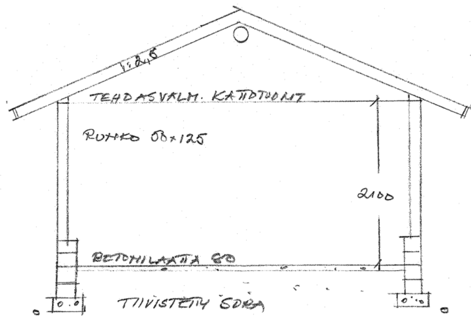
LEIKKAUS A-A
