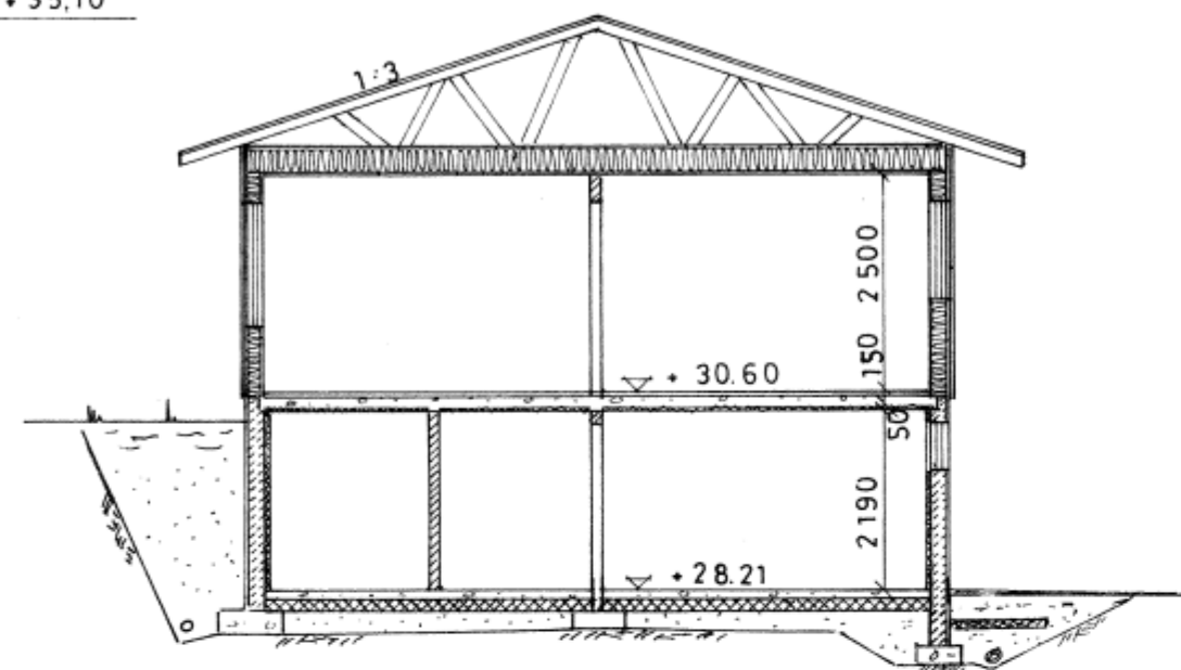
POIKKILEIKKAUS A-A
