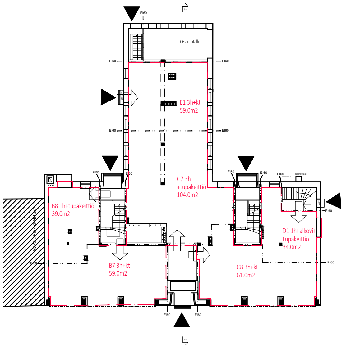
Huoneistotunnisteet ja muutosluerajaus 1:250
