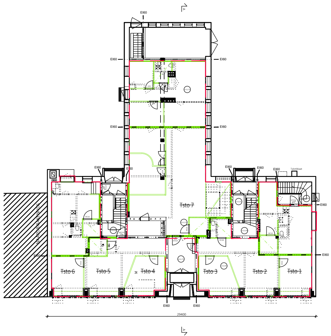
Huoneisto- ja huonejako + purettavat 1:250
