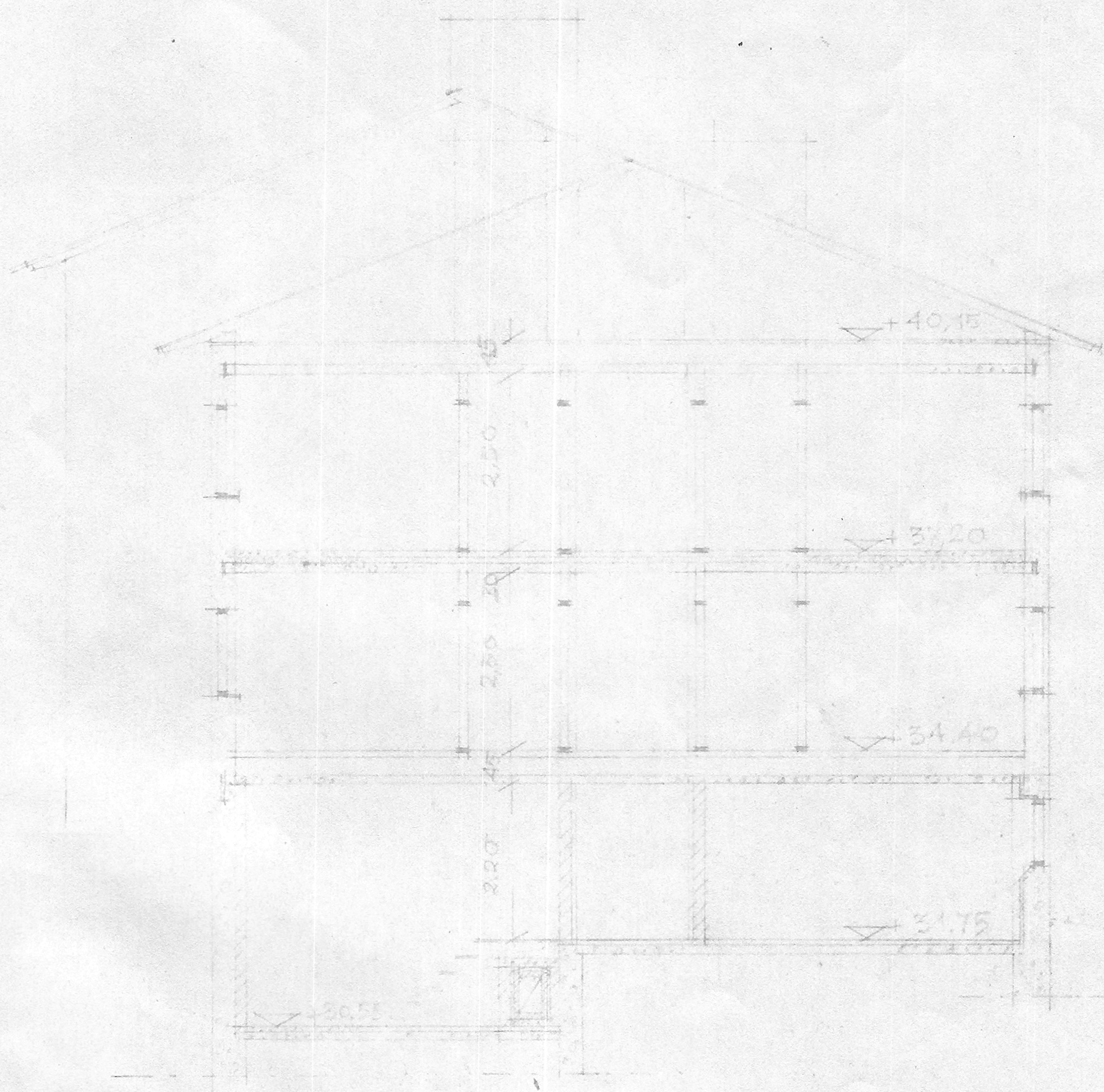
SEKTION A-A
