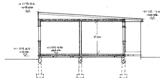
LEIKKAUS A-A 1:100.
