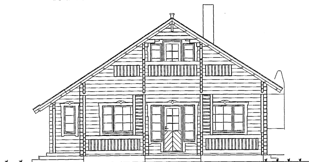
JULKISIVU 1
