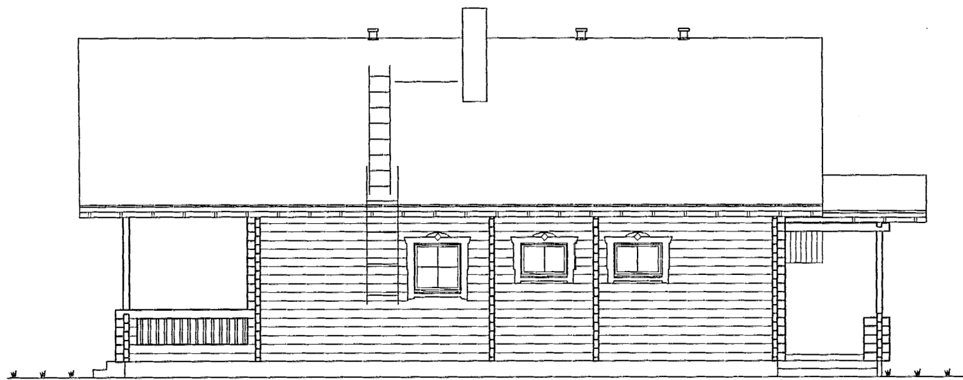
JULKISIVU 2
