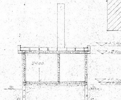
LEIKKAUS A-A
