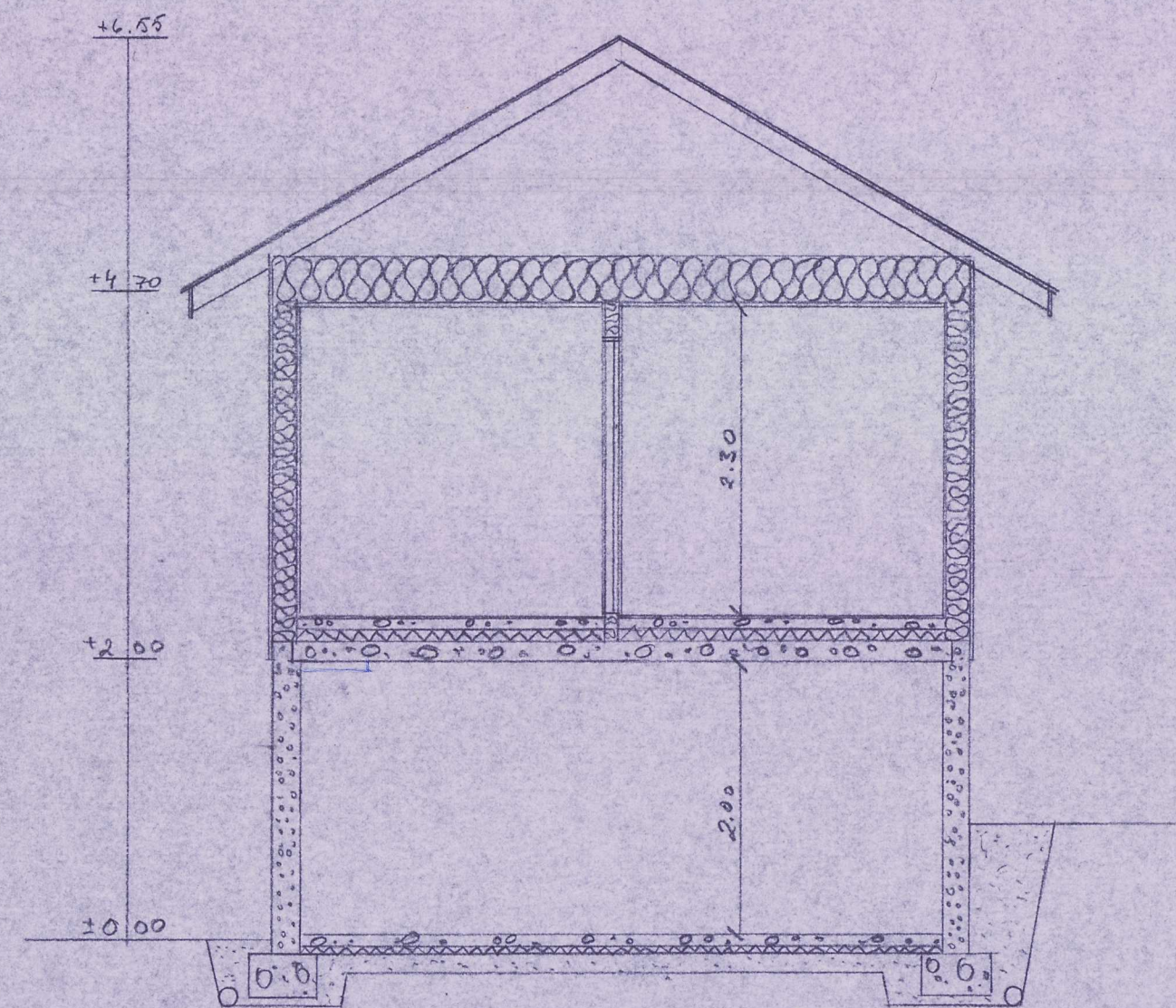
LEIKKAUS A-A
