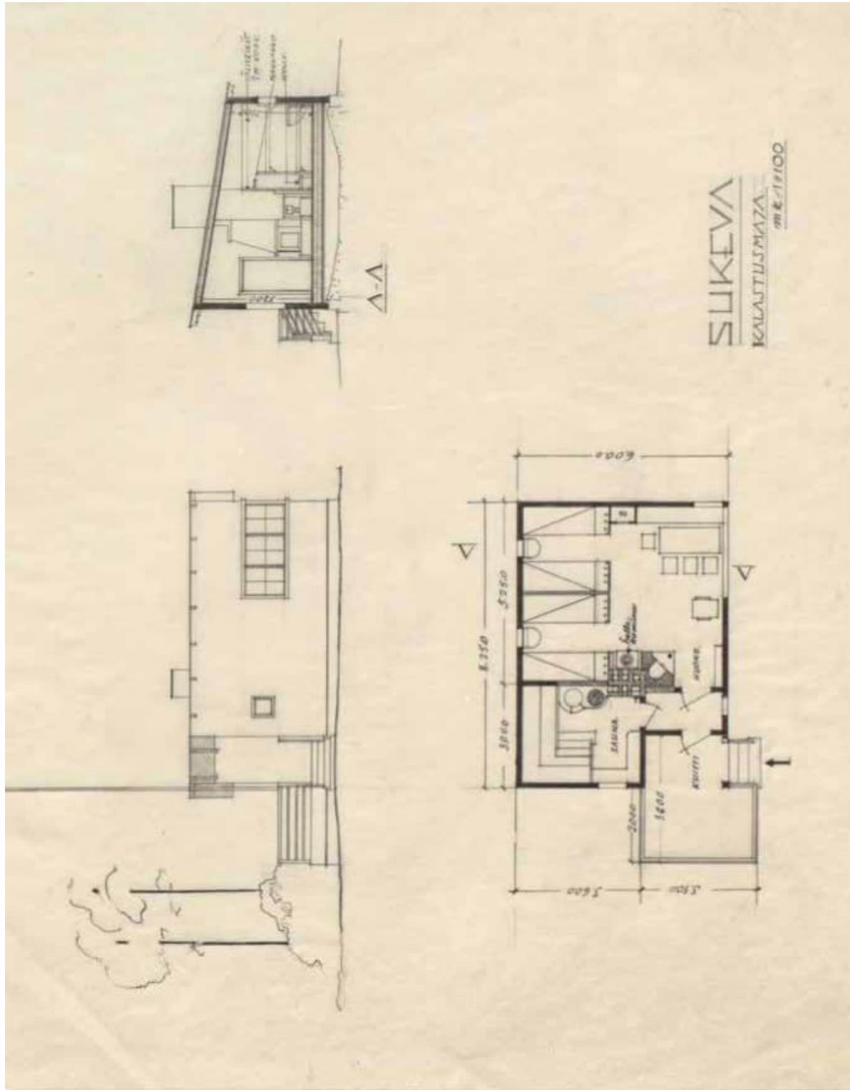
197. Kohteen rakennuspiirustuksia. Suunnitelman laati todennäköisesti arkkitehti Uno Sjöholm 1930-luvulla.
