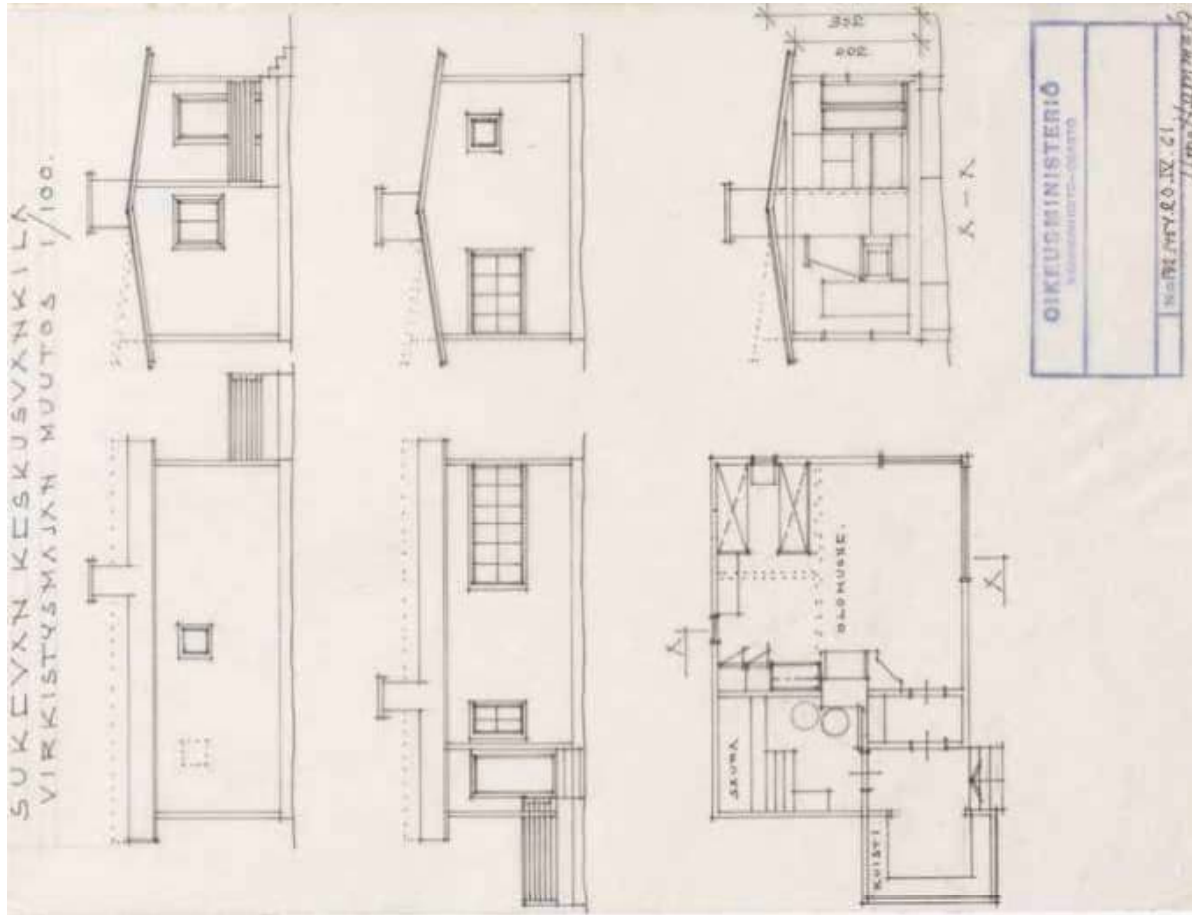
199. Kohteen muutospirustuksia. Suunnitelman laati rakennusmestari Urpo Nummela vuonna 1961.
