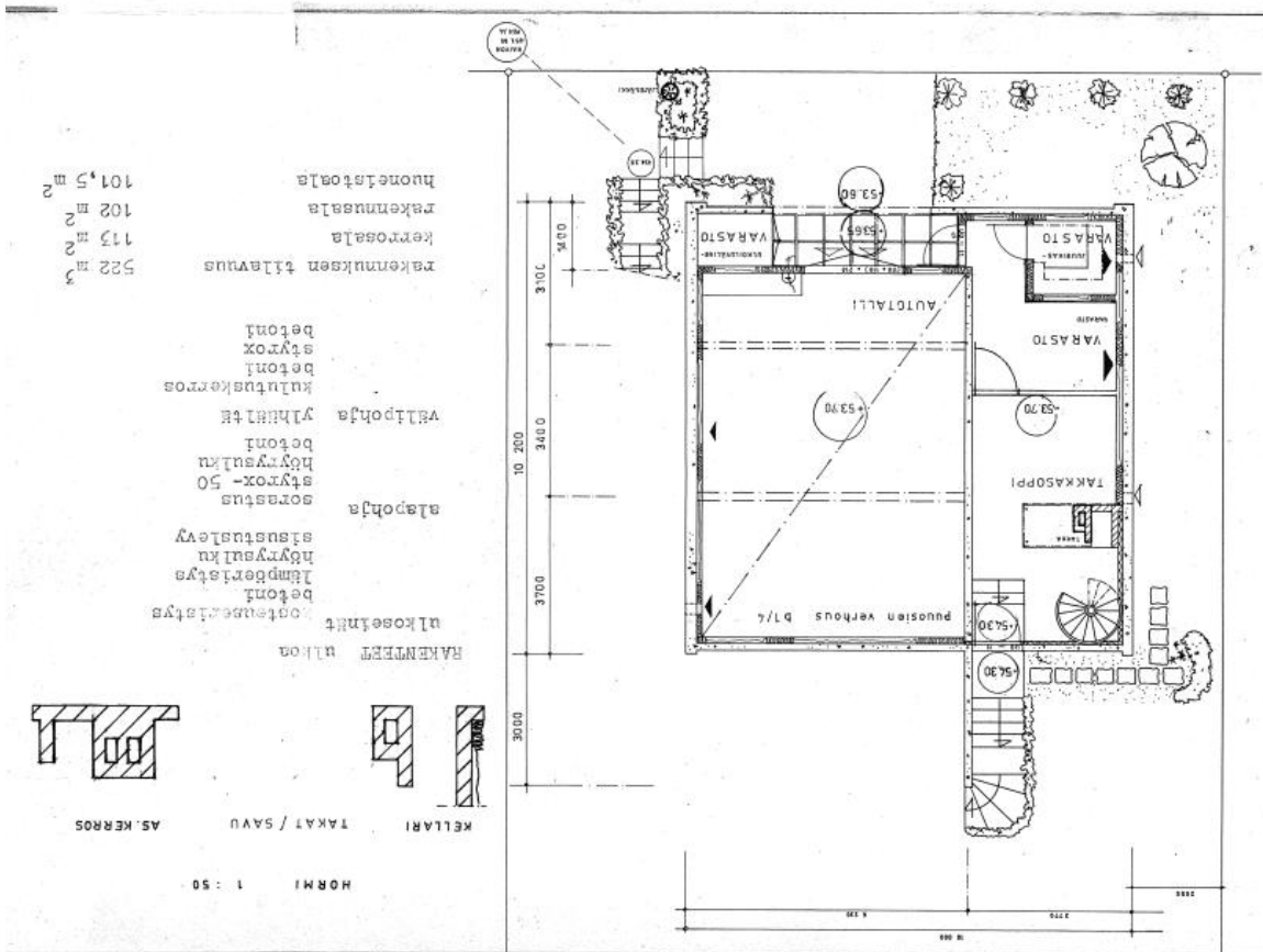
Kellarin pohjakuva. Autotalli muutettu asuinkäyttöön mm. sauna ja pesuhuone on rakennettu alakertaan.
