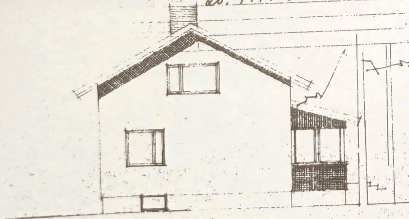
PÄÄTY
