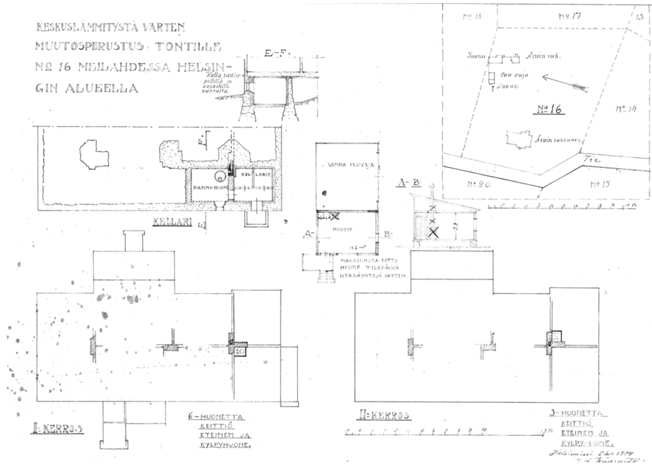
↑ Huvilaan rakennettiin keskuslämmitys 1930-luvulla rakennuksen kellarikerrokseen. Lupapiirustus, elokuu 1934, J.A. Waaranto. HKA.
