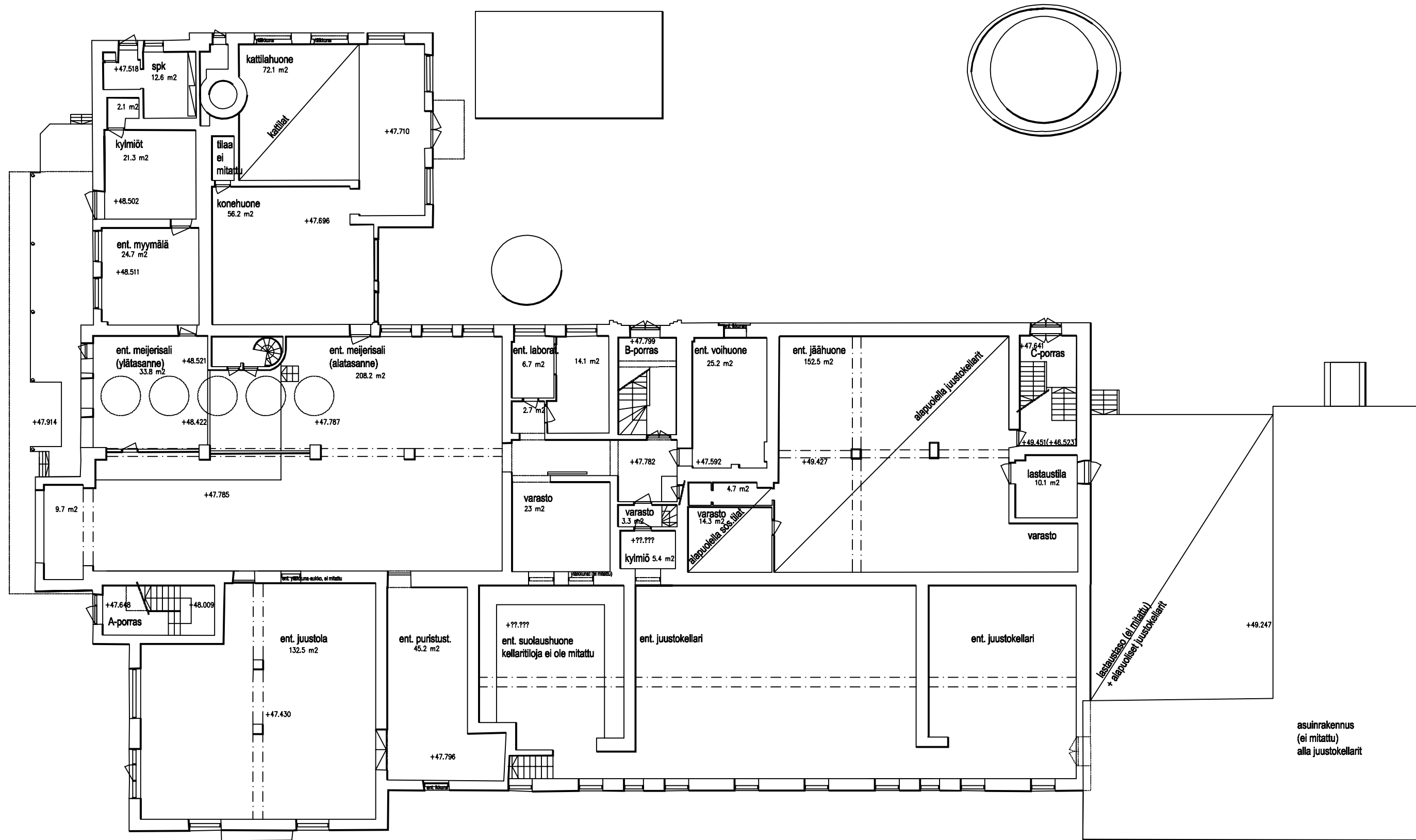
MEIJERI 1.KRS. NYKYTILANNE maaliskuu 2006 Tilojen päämitat ja korkotasotiedot mitattu ja päivitetty piirustuksiin. Mitat tarkistettava paikalta!
