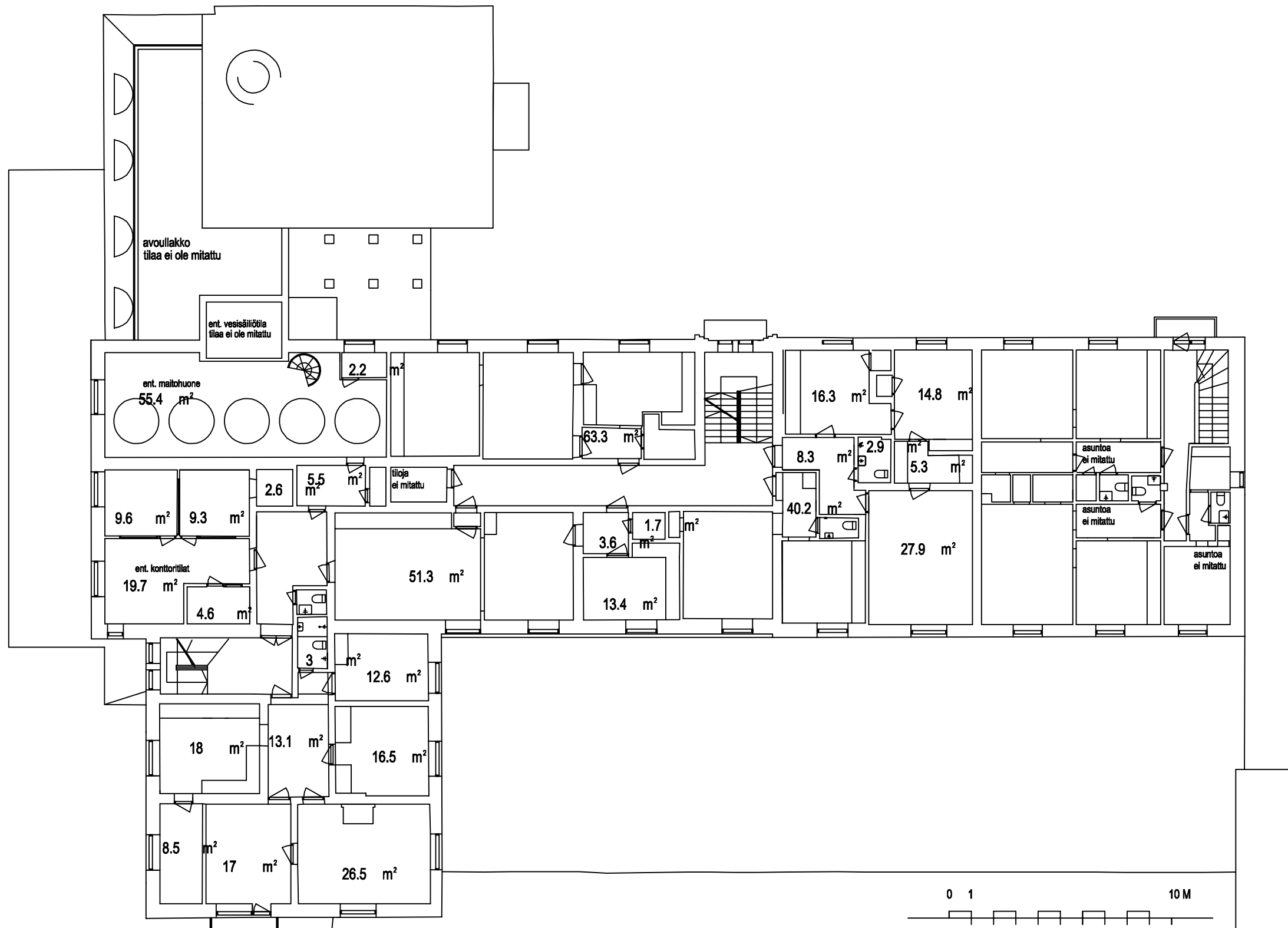
MEIJERI 2.KRS. NYKYTILANNE maaliskuu 2006 Tilojen päämitat ja korkotasotiedot mitattu ja päivitetty piirustuksiin. Mitat tarkistettava paikalta!
