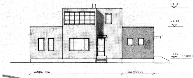
JULKISIVU ETELÄÄN
