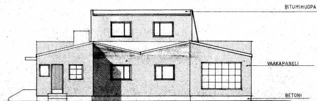
JULKISIVU PÖHJOISEEN
