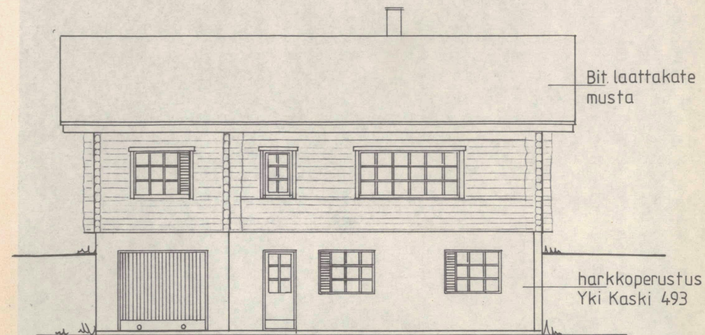
JULKISIVU LÄNTEEN
