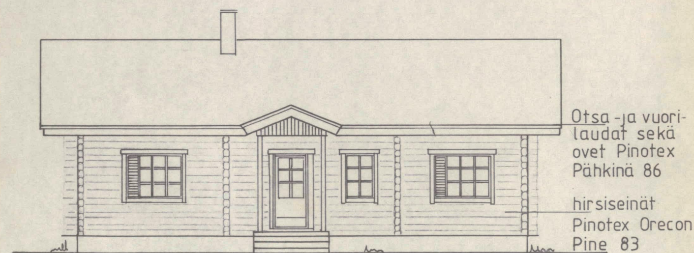
JULKISIVU ITÄÄN
