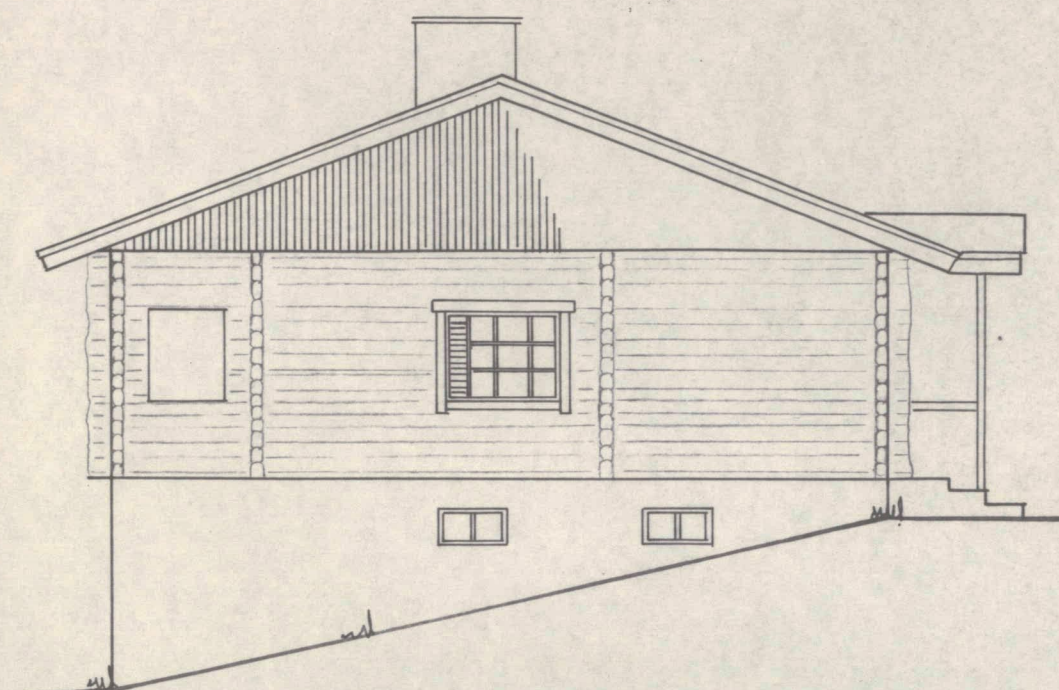
PÄÄTY ETELÄÄN
