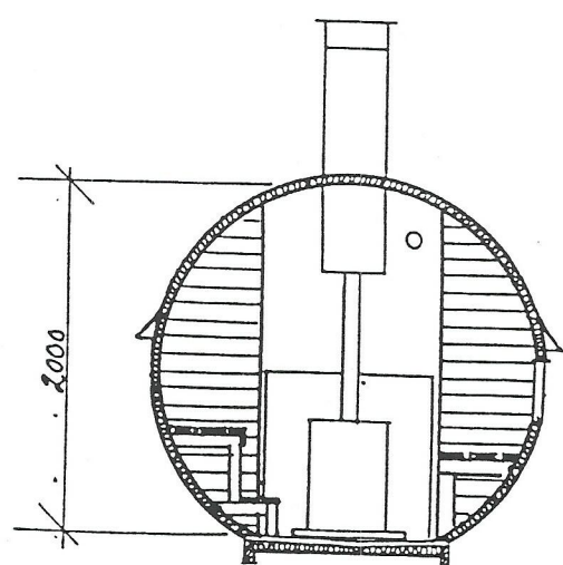
LEIKKAUS Q-Q
