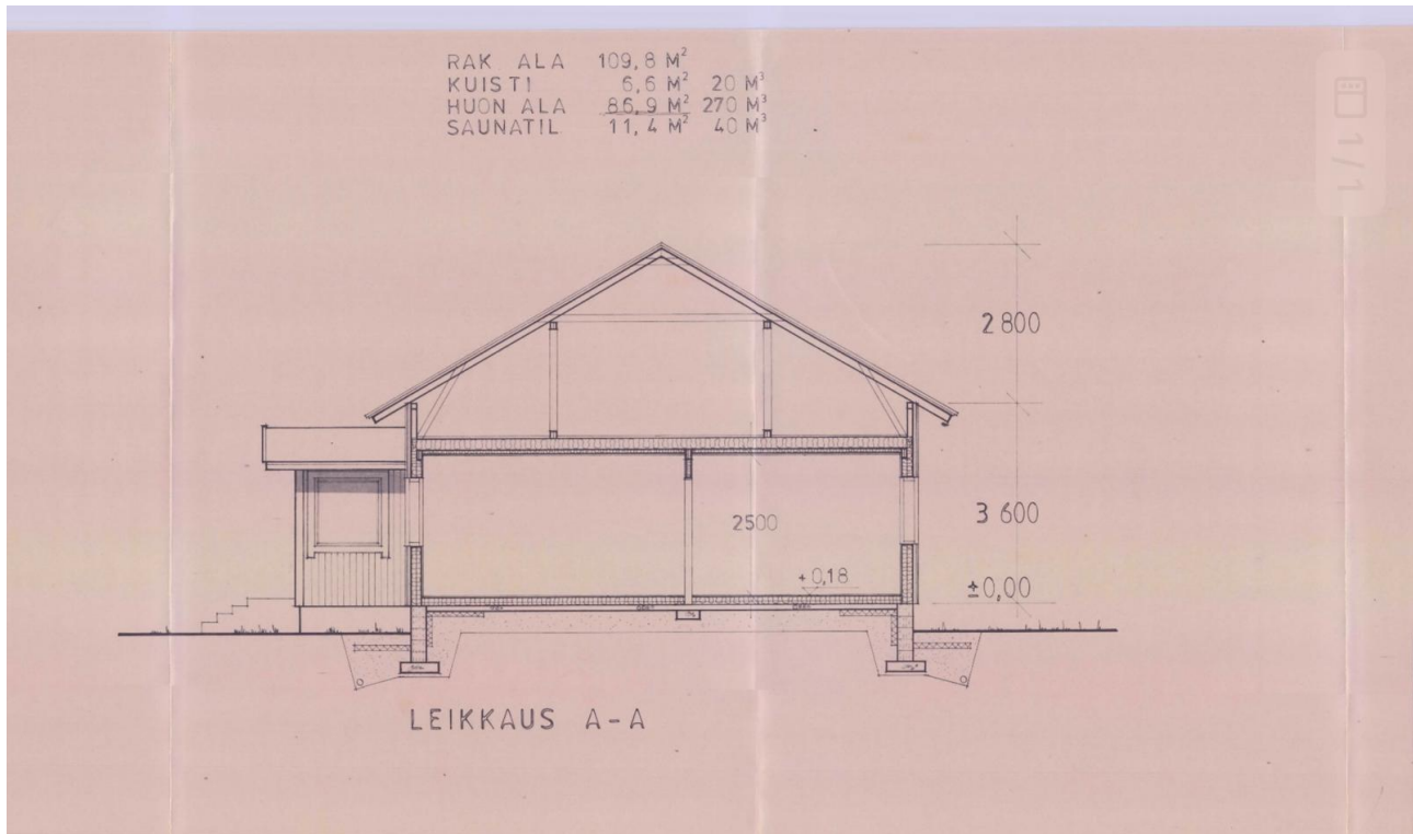
Leikkauskuva
