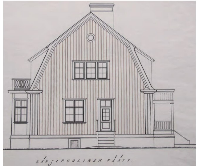
Julkisivu länteen.
