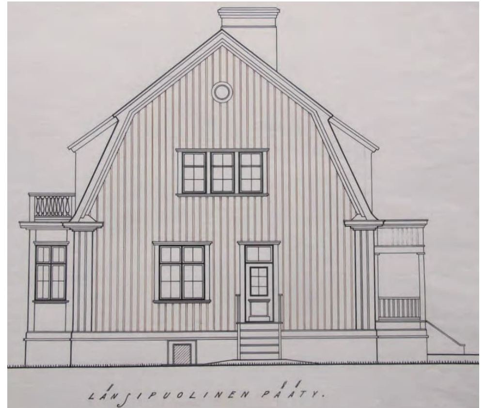
Julkisivu länteen.
