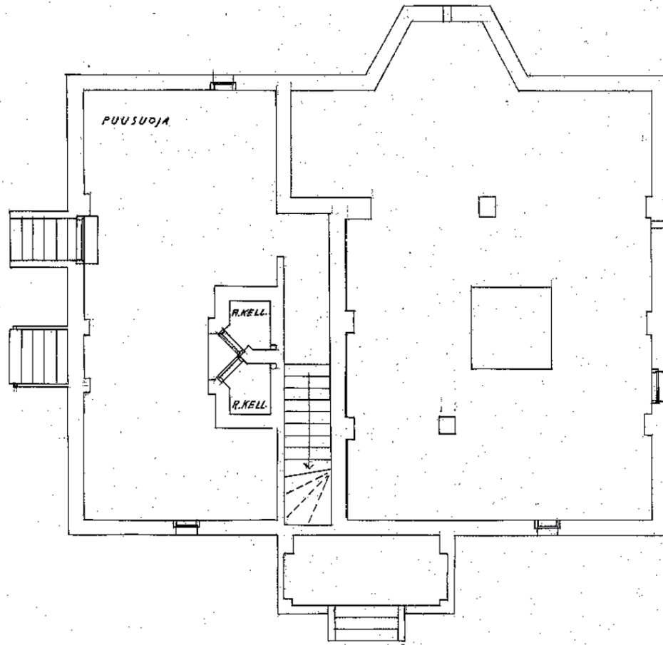
Kellarin pohjapiirros.
