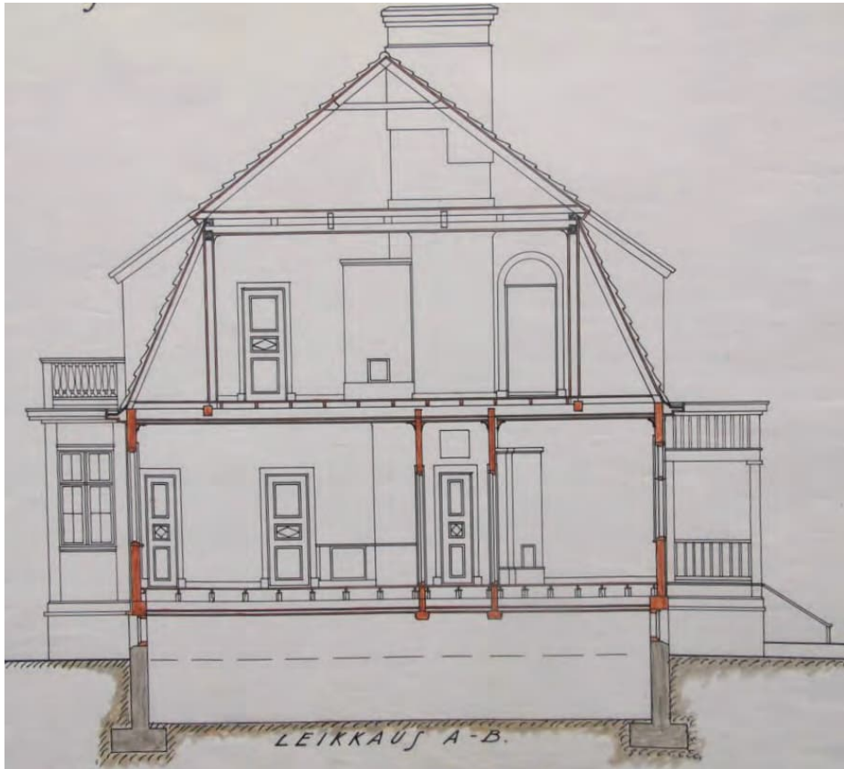
Leikkaus.
