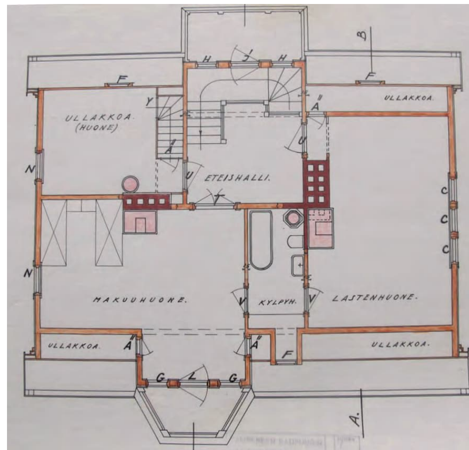
Ullakkokerroksen pohjapiirros.
