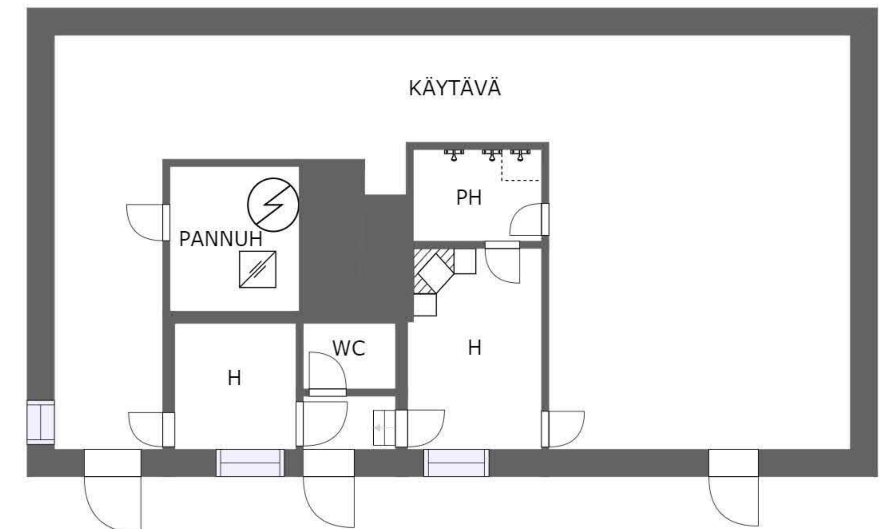
KELLARIKERROS
