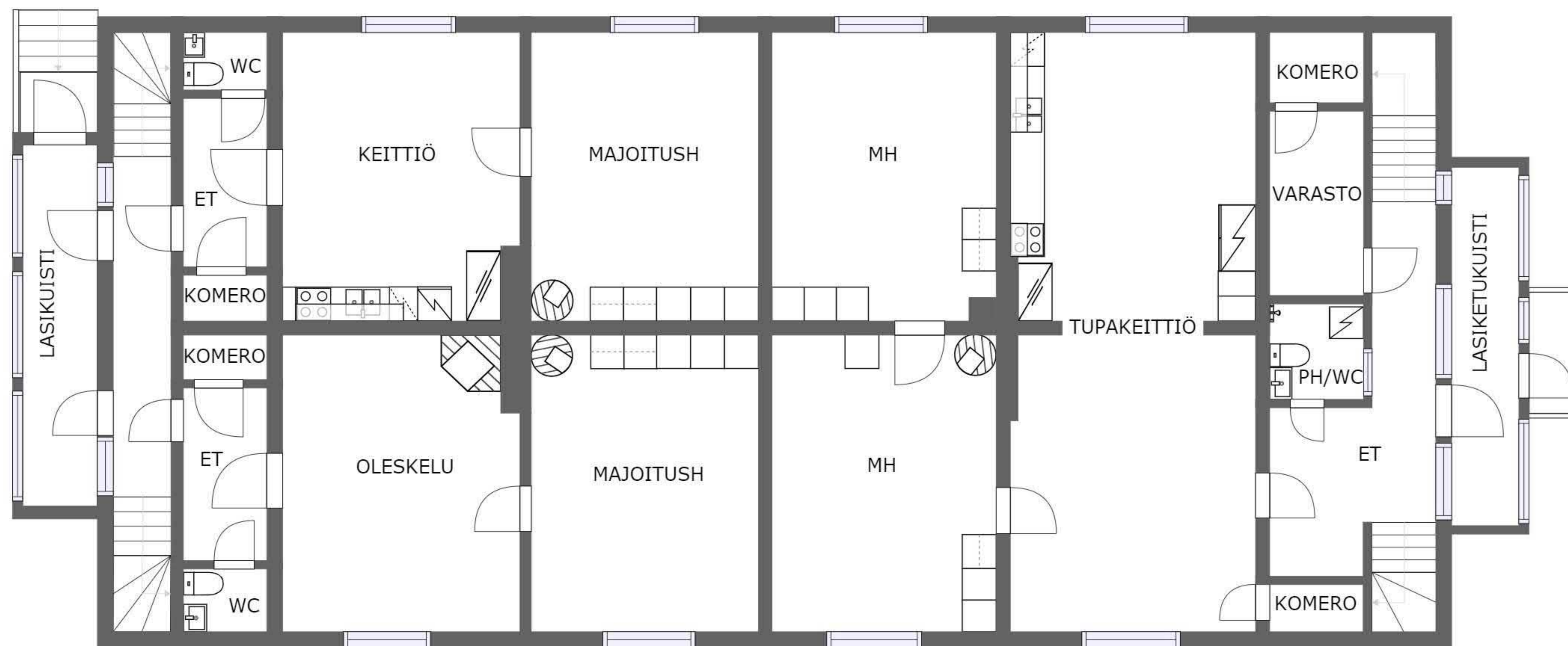
1. KERROS
