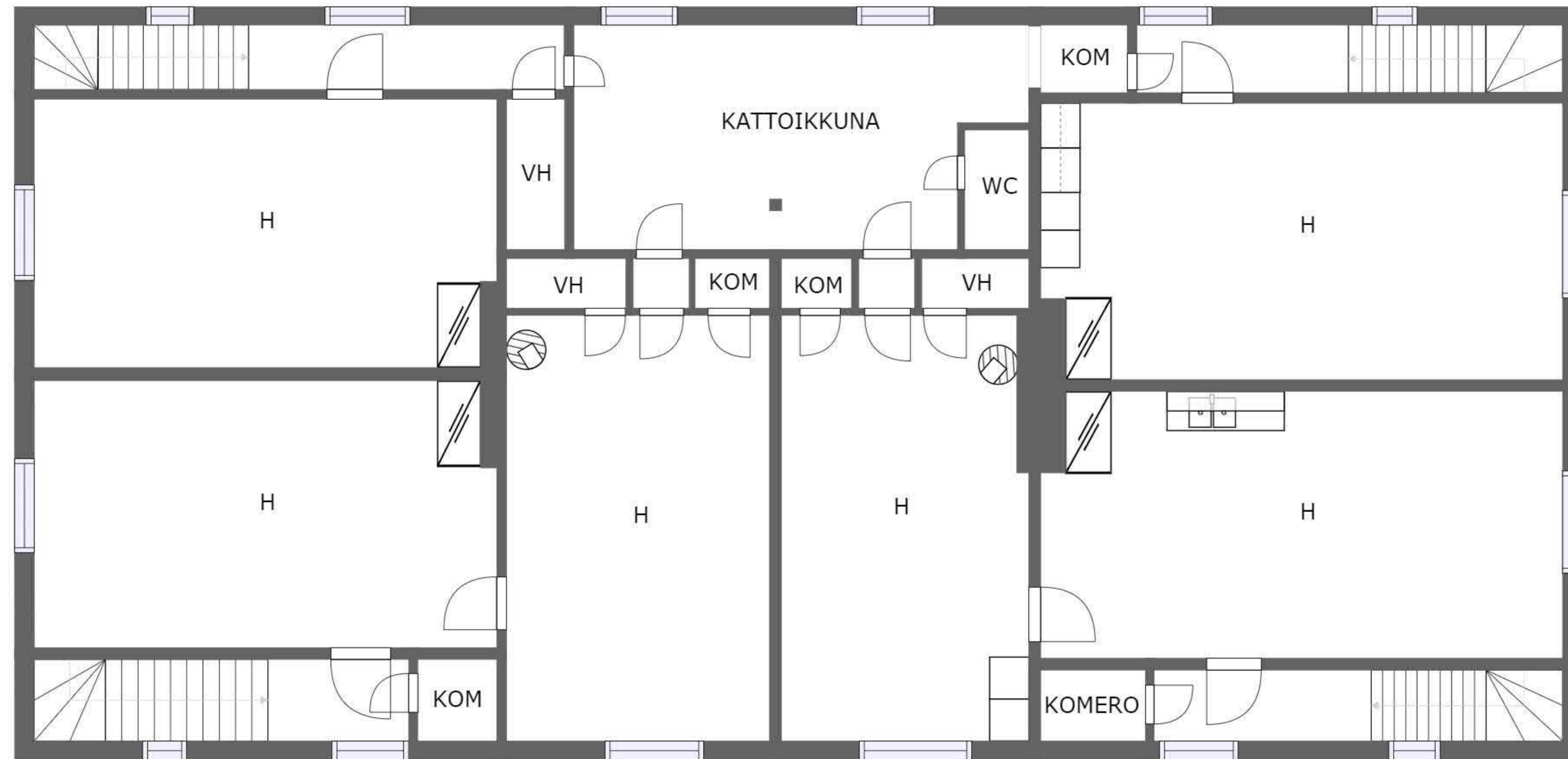
2. KERROS
